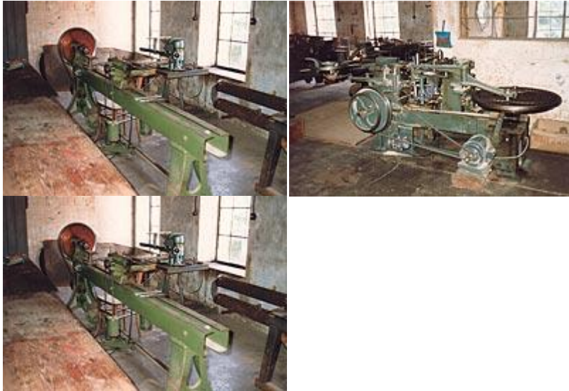
Machines pour manufacture de brosses (Collection: Georges Ginter)
