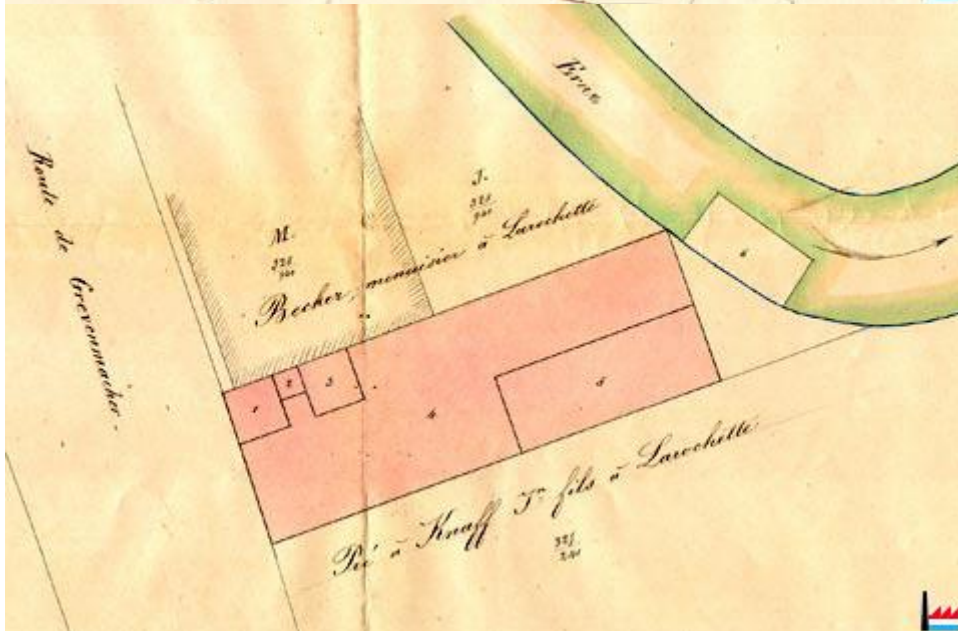
Plan de la Teinturerie et lavoirs à laine Jean et Charles Knaff à construire à l'entrée de Larochette, au lieu dit "Platzwies" aux abords de la route de Larochette à Graulinsten - 1876
