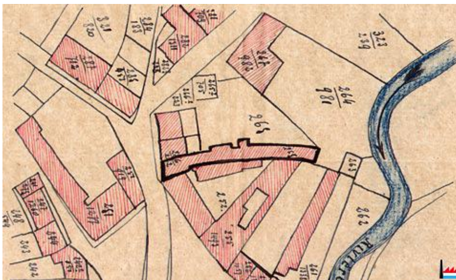
Fabrique Edgar Delmarque, Larochette - 1920 (Document: ANLux )
