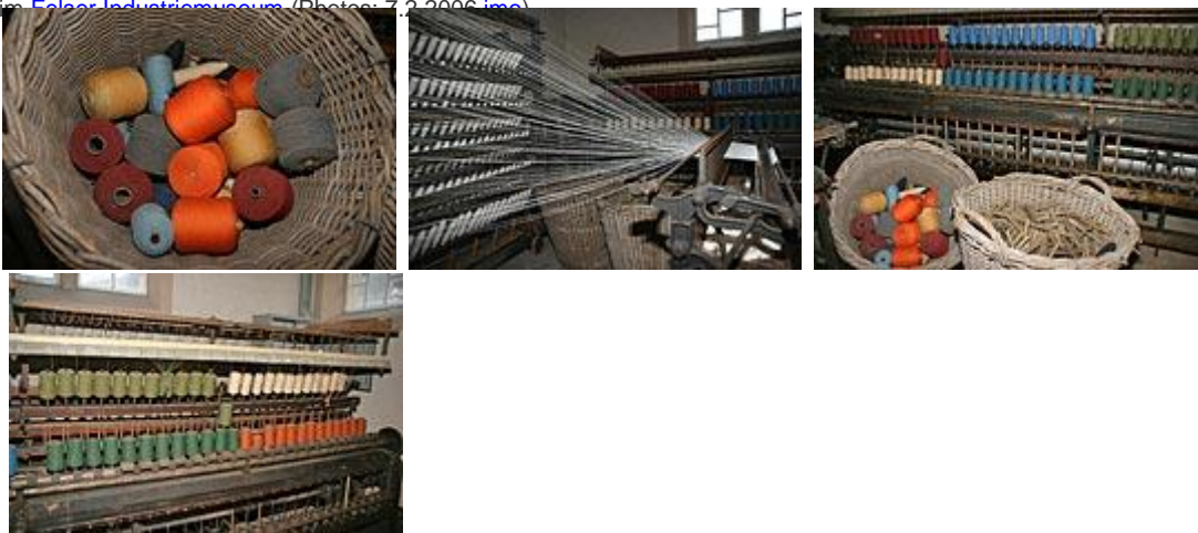
Retordeuse Thieron de la Draperies de Larochette au Musée industriel à Larochette Thieron Zwirnerei Maschine der Draperies de Larochette im Felser Industriemuseum (Photos: 7.2.2006 jmo )
